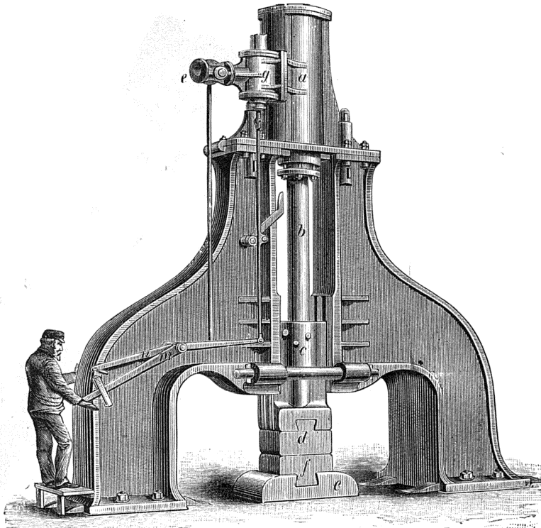
1. Молотъ Massey съ двумя ногами.
