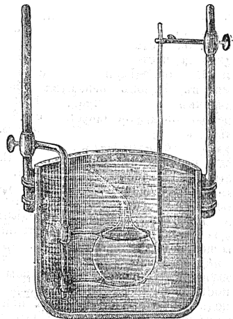
Фиг. 3. Приборъ Дюма.
