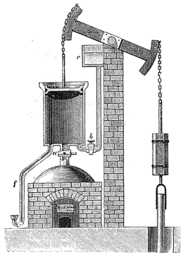
3. Машина Ньюкомена и Коудера.
