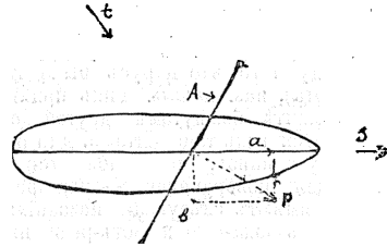
A — плоскость паруса; P — давленіе ветра на парусъ; s — курсъ судна; t — направленіе ветра; a и b — см. въ текстѣ.
