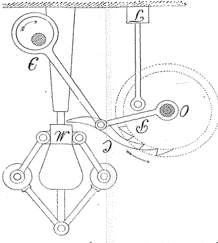
Фиг. 5 Разновидности цилиндрической машины
