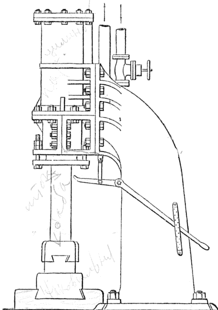
2. Молотъ съ толстымъ штокомъ типа Морисона.
