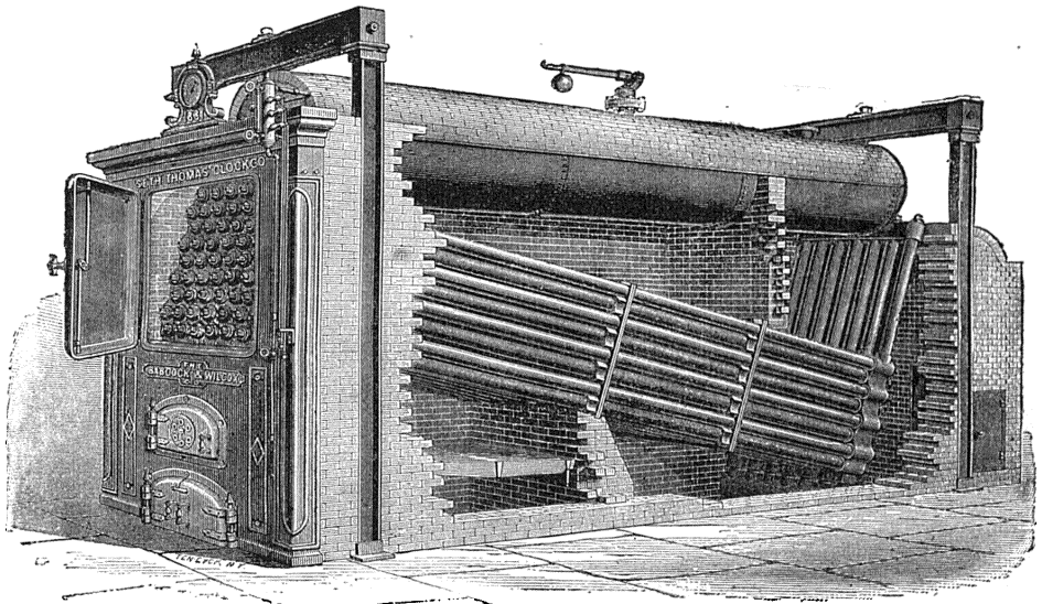
Черт. 7. Водотрубный котель Бабкока и Вилькокса.
