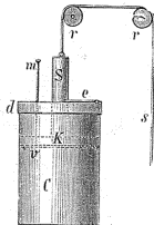
1. Прибор Палепа
