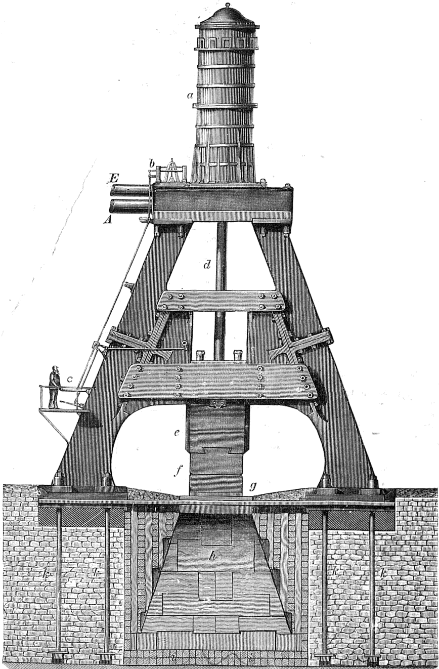
3. Молотъ въ желѣзодѣлательномъ заводѣ въ Кресо.
