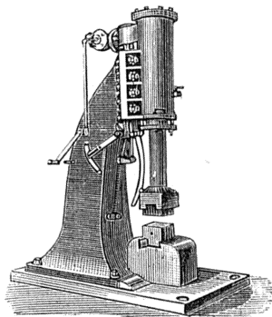
3. Молотъ Massey типа Морисона съ одной станиной.
