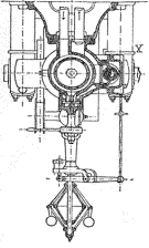
Фиг. 6 Паровая машина с двойным давлением пара
