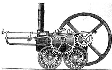
2. Паровоз Тревиттика (1801).
