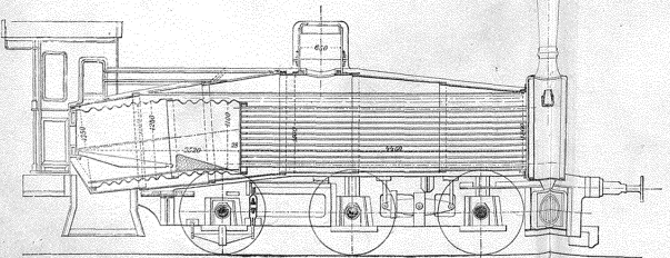
Черт. 5. Товарный паровоз с котлом Ленца (Lentz).
