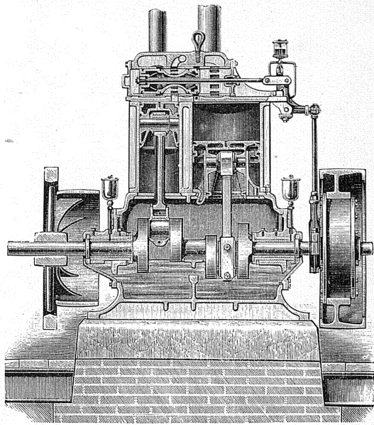
Быстроходная паровая машина колланульд Вестингауза.
