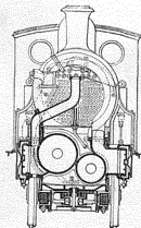
Черт. 6. Котел уэльс-паровоз. Вортелла (Wortell).
