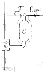
2. Машина Савери.
