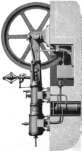
2. Горизонтальная паровая машина Вульфа.
