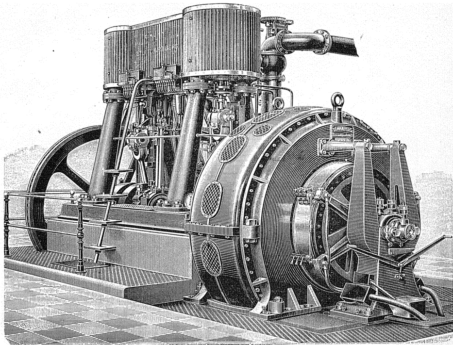
Вертикальная паровая машина компаундъ съ динамо-машиной.
