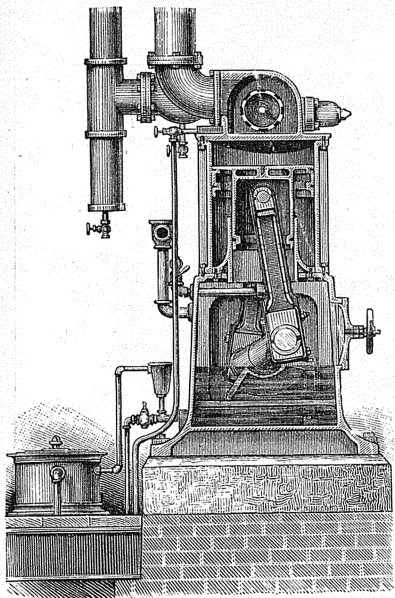
Быстроходная паровая машина колланульд Вестингауза.
