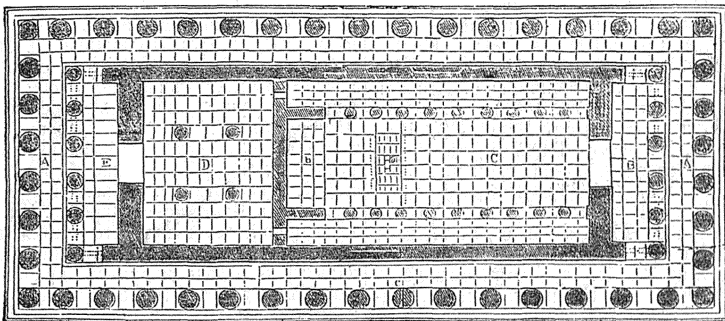
Фиг. 2. Планъ Парфенона.
