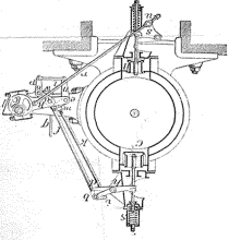
Фиг. 10. Паровая цилиндрическая машина
